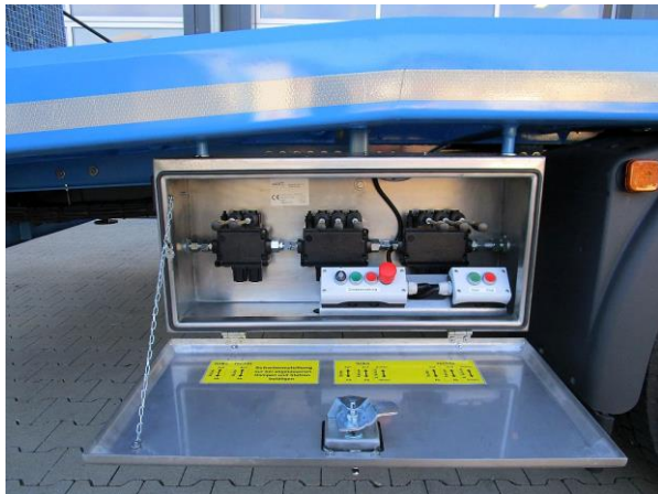
hydr. Abstützung m. bewegl. Teller
